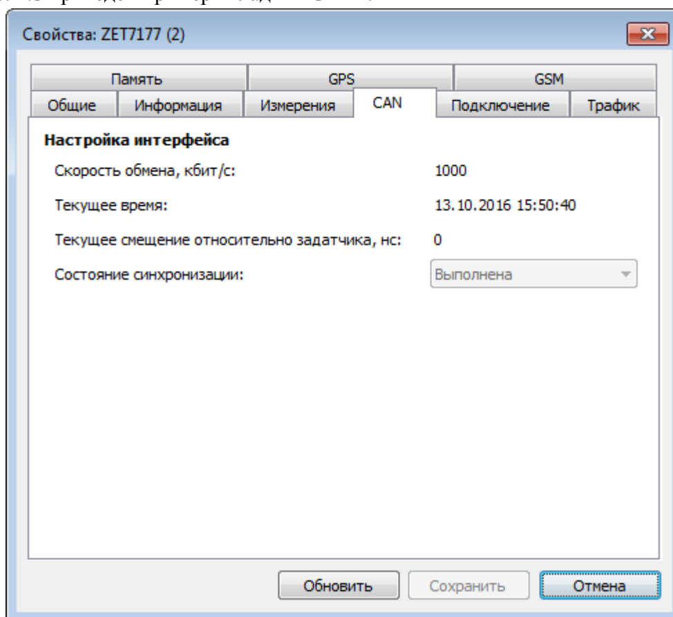
Рис. 4.3 Вкладка «CAN»
