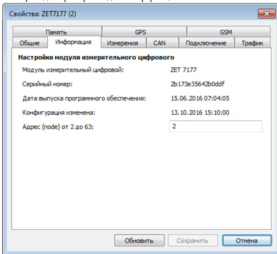
Рис. 4.2 Вкладка «Информация»
