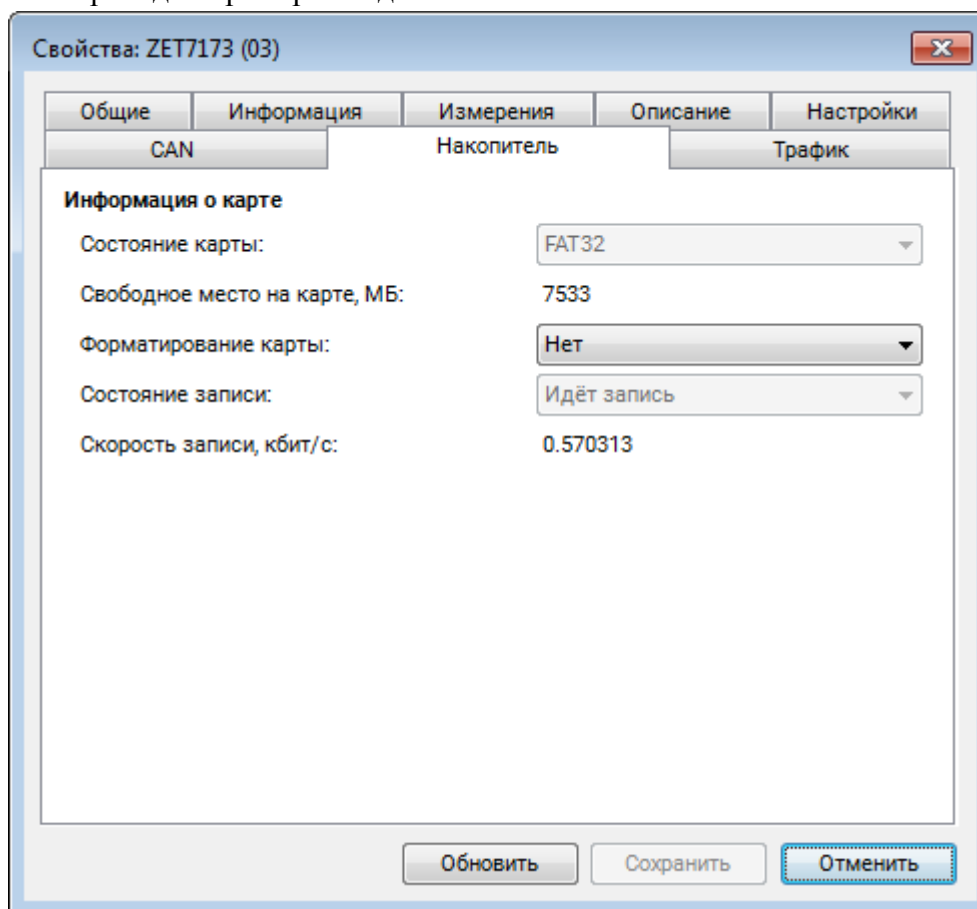
Рис. 4.3 Вкладка «Накопитель»
